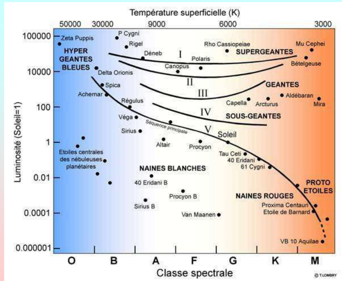
Diagramme H-R : température - luminosité.
